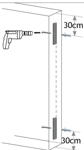
Fissaggio con aletta
